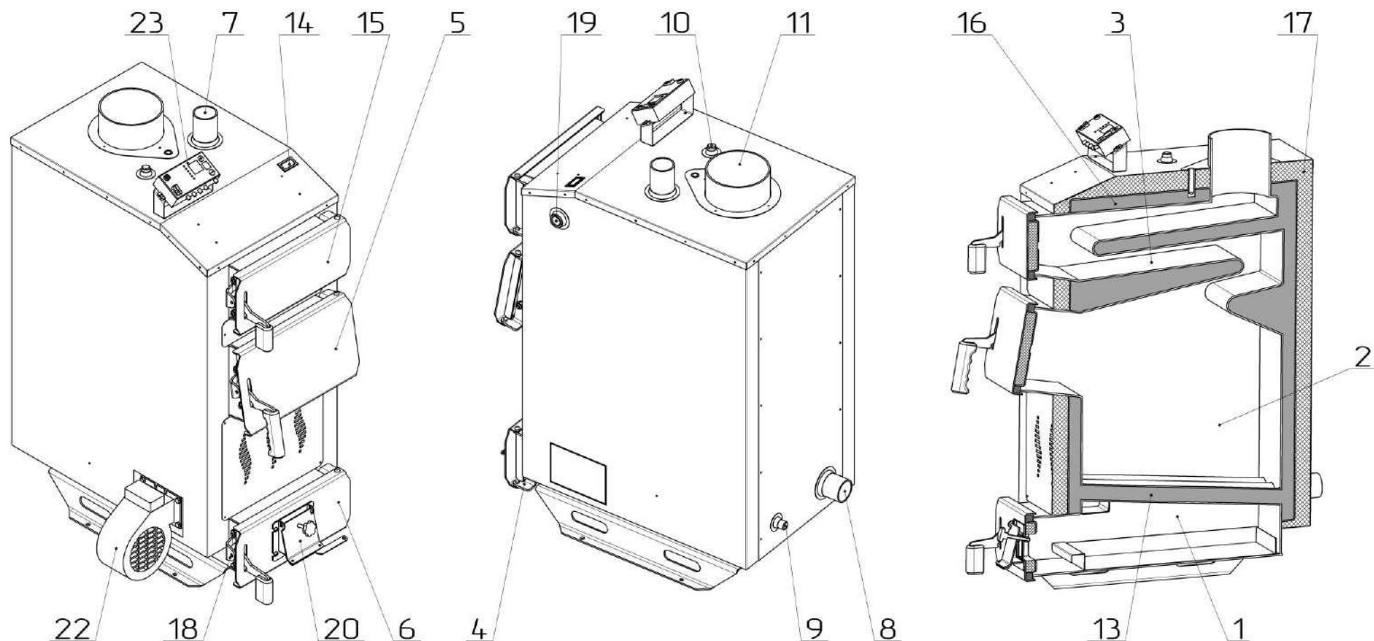
Рисунок 2б – Внешний вид и основные элементы котла Praktik Plus
