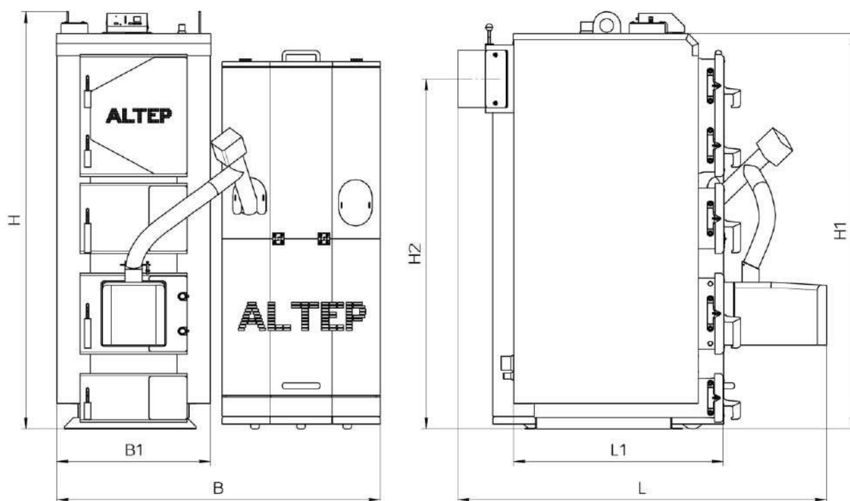
Рисунок 1 – Габаритный чертеж котла типа КТ-2Е-РG
