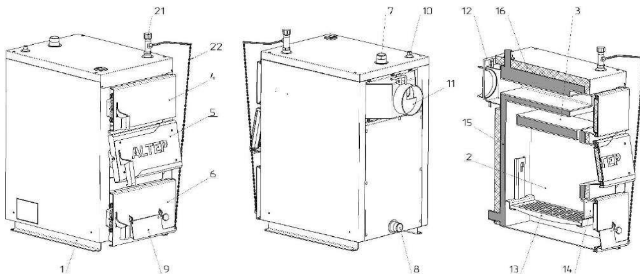
Рисунок 2 - Основные элементы котла Alter-Компакт
